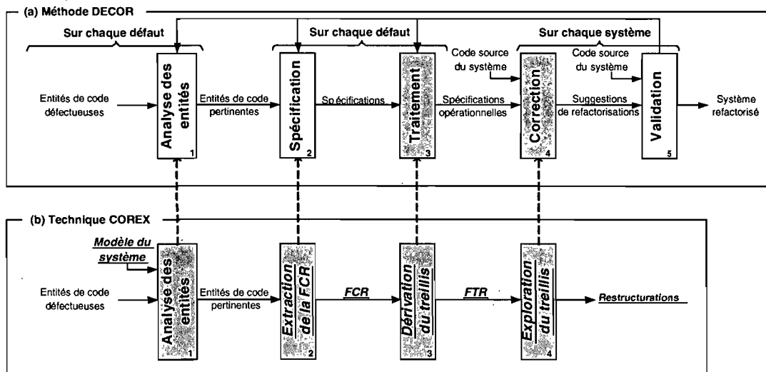
FIG. 4.5 – (a) La méthode DECOR. (b) La technique de correction COREX (les étapes, entrées et sorties en gras, italiques et soulignés sont spécifiques à COREX en comparaison avec DECOR).
