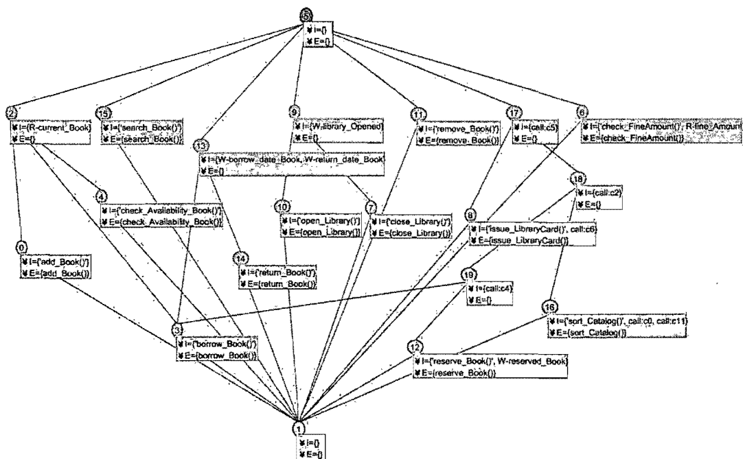
FIG. 4.7 – Treillis associé au contexte de la figure 4.6.
