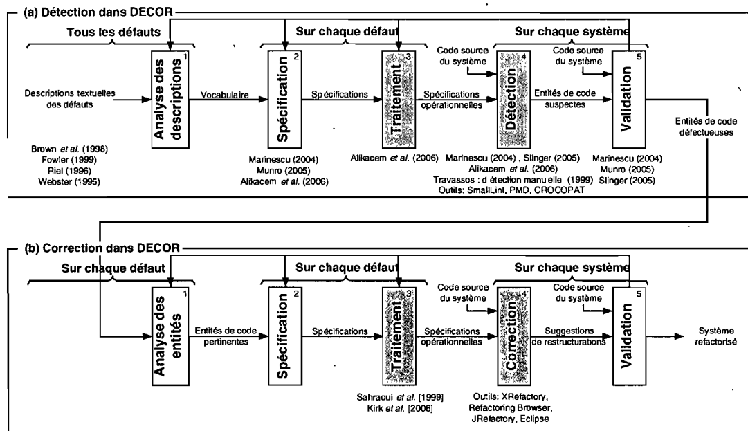
FIG. 2.2 – La méthode DECOR comparée aux travaux liés.
