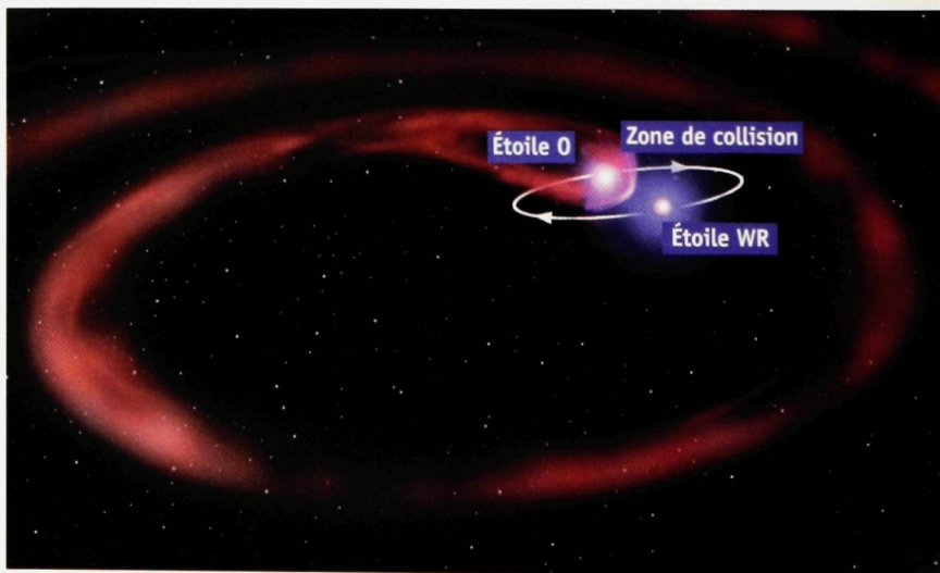
Reconstitution de la spirale de particules de carbone formées dans la zone de collision des vents solaires d'une étoile double. L'étoile Wolf-Rayet (WR) est plus massive et possède un vent plus puissant que sa compagne de type 0.
