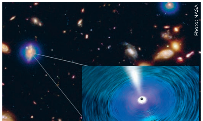
Illustration d'un trou noir « ultramassif » détecté par les chercheurs.
