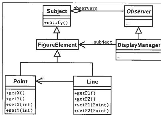
FIG. 1.3: Exemple FigureElement : utilisation du patron Observer
