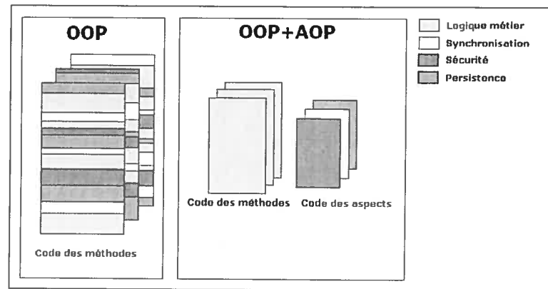
FIG. 1.1: Encapsulation des préoccupations transversales
