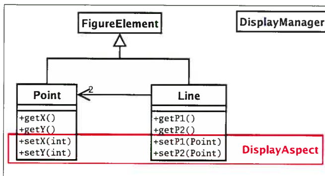
FIG. 1.4: Exemple FigureElement : approche orientée aspect
