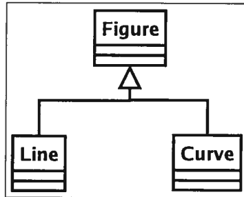
FIG. 2.3: DIT : hiérarchie originale
