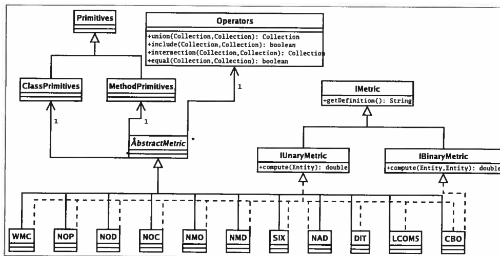
FIG. 3.4: Architecture simplifiée de la bibliothèque POM
