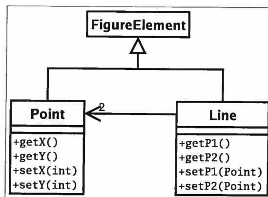
FIG. 1.2: Exemple FigureElement
