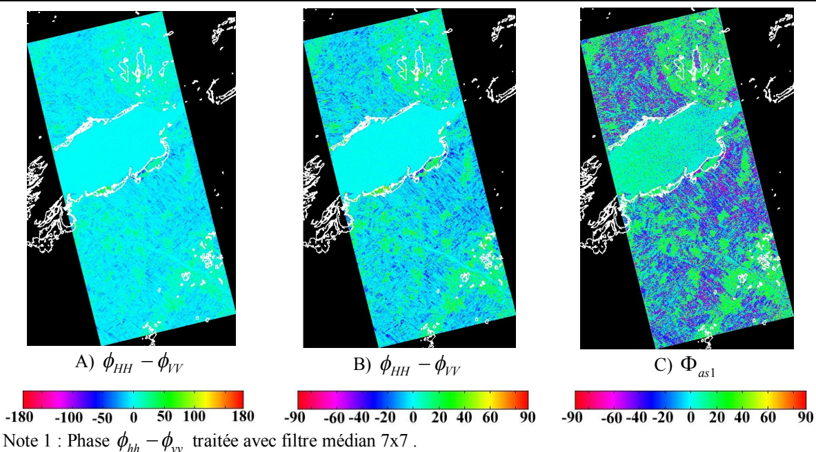
Figure 10.3-1 : Images des phases \phi_{hh} - \phi_{vv} et de \Phi_{\alpha s1} (novembre 2006)
