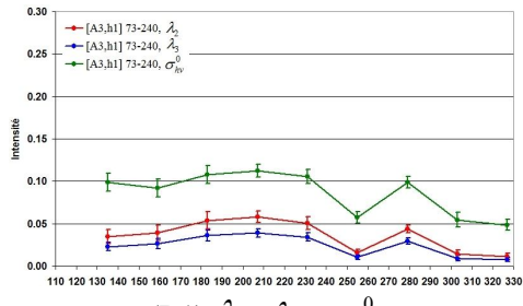
(D1) \lambda_2 , \lambda_3 et \sigma_{hv}^0
