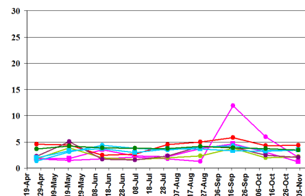
(L) |\psi_1|
