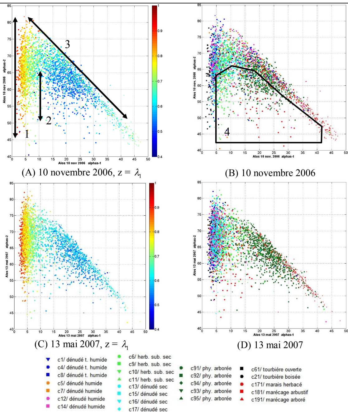
Figure 10.5-1 : Relation entre le type dominant ( \alpha_{s1} ) et le second type de rétrodiffusion symétrique ( \alpha_{s2} ) par classe physiologique selon \lambda_{1N} , 10 novembre 2006 et 13 mai 2007
