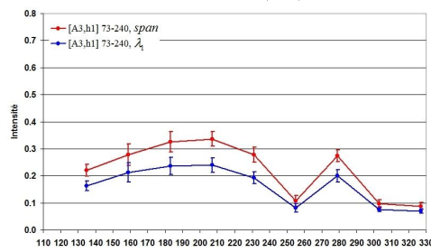
(C1) span et \lambda_1
