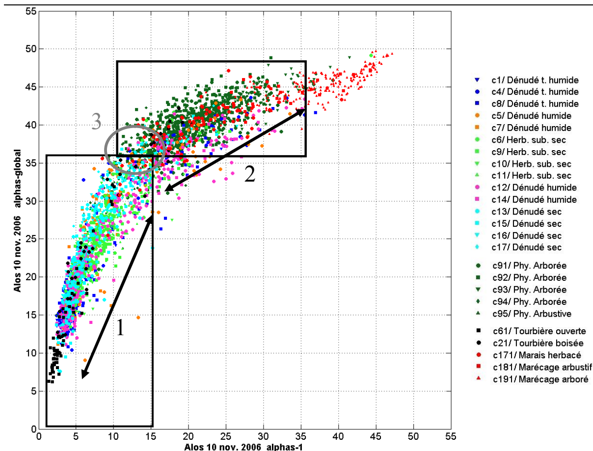
Figure 10.5-5 : Relation entre le type dominant de rétrodiffusion symétrique ( \alpha_{s1} ) et le type global de rétrodiffusion symétrique ( \alpha_{sg} ), par physiologie végétale, 10 novembre 2006
