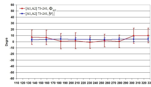
(B2) \Phi_{\alpha_{s1}} et |\psi_1|
