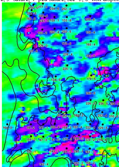
(D) Alos-Palsar, 2007-05-13, \Phi_{\alpha s1} (conditions sèches)
