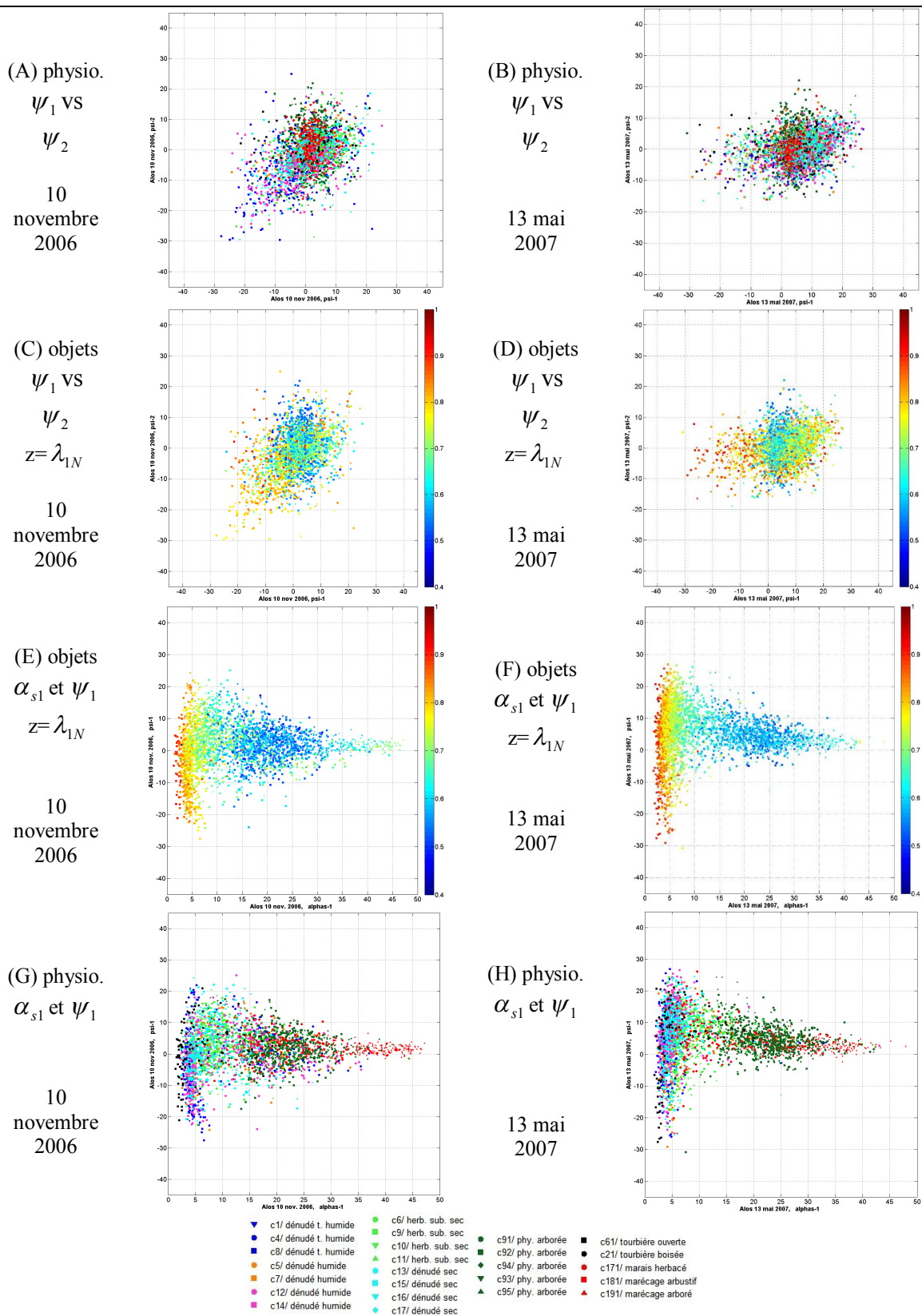
Figure 10.7-3 : Relation entre le premier ( \psi_1 ) et second ( \psi_2 ) angle d'orientation par classe physionomique et en fonction de \lambda_{1N} et \alpha_{s1}
