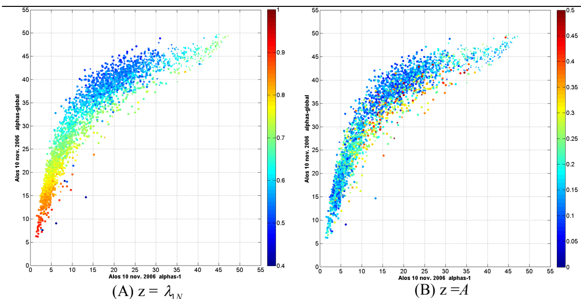
Figure 10.5-6 : Relation entre le type dominant de rétrodiffusion symétrique ( \alpha_{s1} ) et le type global de rétrodiffusion symétrique ( \alpha_{sg} ), en fonction de la première valeur propre ( \lambda_{1N} ) et de l'anisotropie ( A ), 10 novembre 2006
