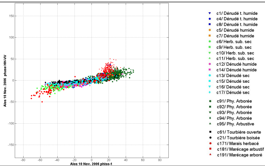
Figure 10.3-2 : Comparaison entre \phi_{hh} - \phi_{vv} et \Phi_{\alpha s1} par classe phytosociologique
