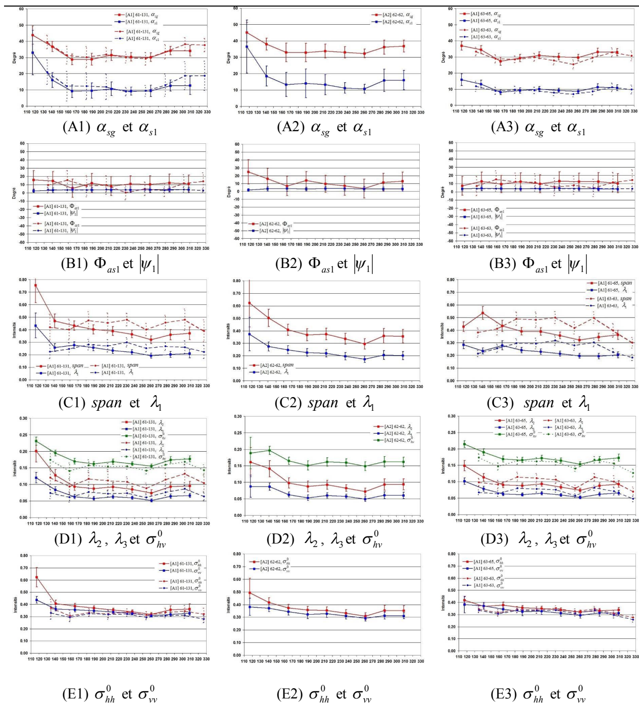
Figure 12.3-1 : Signatures saisonnières des marécages arborés [A1-131] (1 ère col.); marécages arbustifs [A2-62] (2 e col.) et des physiognomies arborées sur substrat sec [A1-63&65] (3 e col.). Séries FQ15-A (trait plein) et FQ21-D (trait pointillé)
