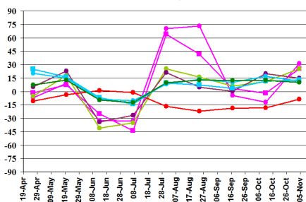
(J) \Phi_{\alpha_{s1}}
