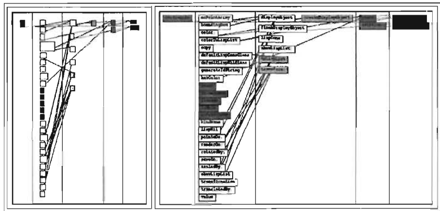
FIG. 2.7 – Visualisation blueprint d'une classe par Ducasse et Lanza [8].
