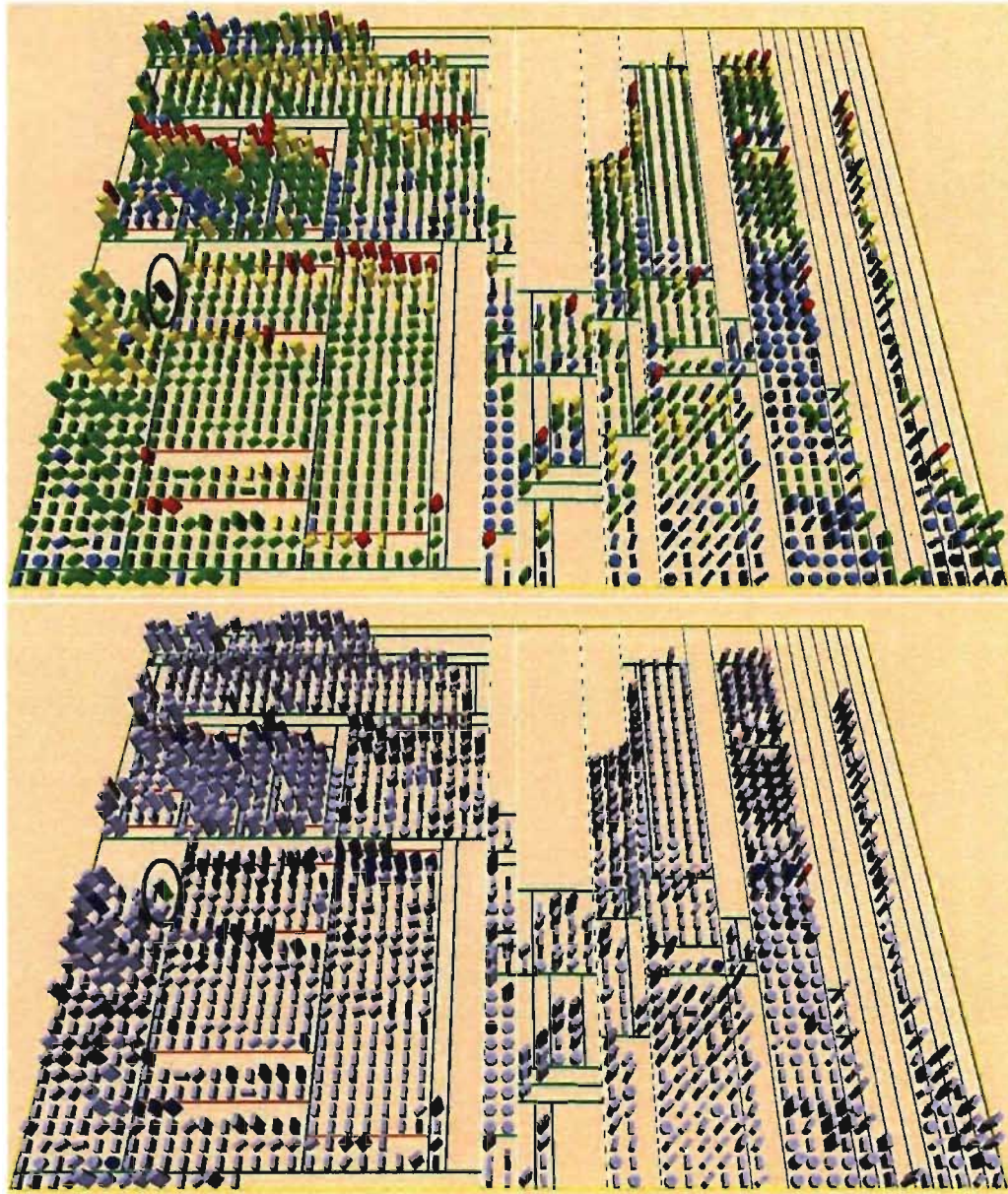
FIG. 5.5 – Un exemple de symptôme de changement divergeant trouvé dans ArgoUML . (Haut) Filtre de distribution appliqué sur NUC. (Bas) Filtre d'associations appliqué sur la classe encerclée.
