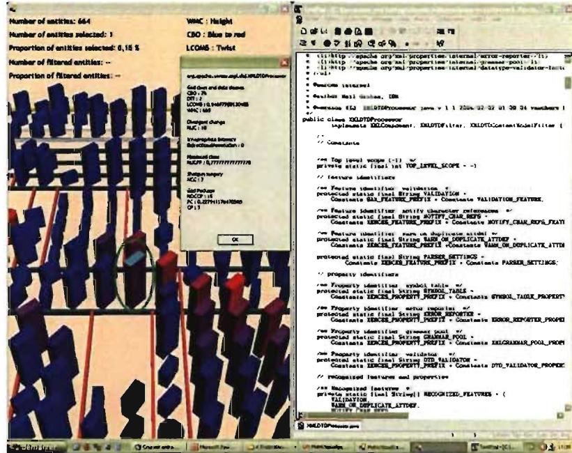
FIG. 4.16 – Accès au code source d'une classe à partir de VERSO.
