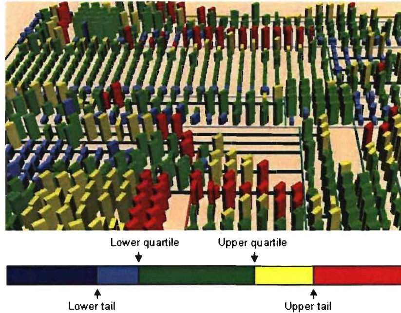
FIG. 4.3 – Une vue de Xerces avec le filtre de distribution appliqué pour la métrique CBO.
