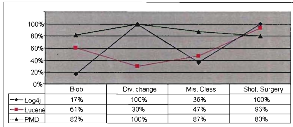
FIG. 6.2 – Précisions par système.
