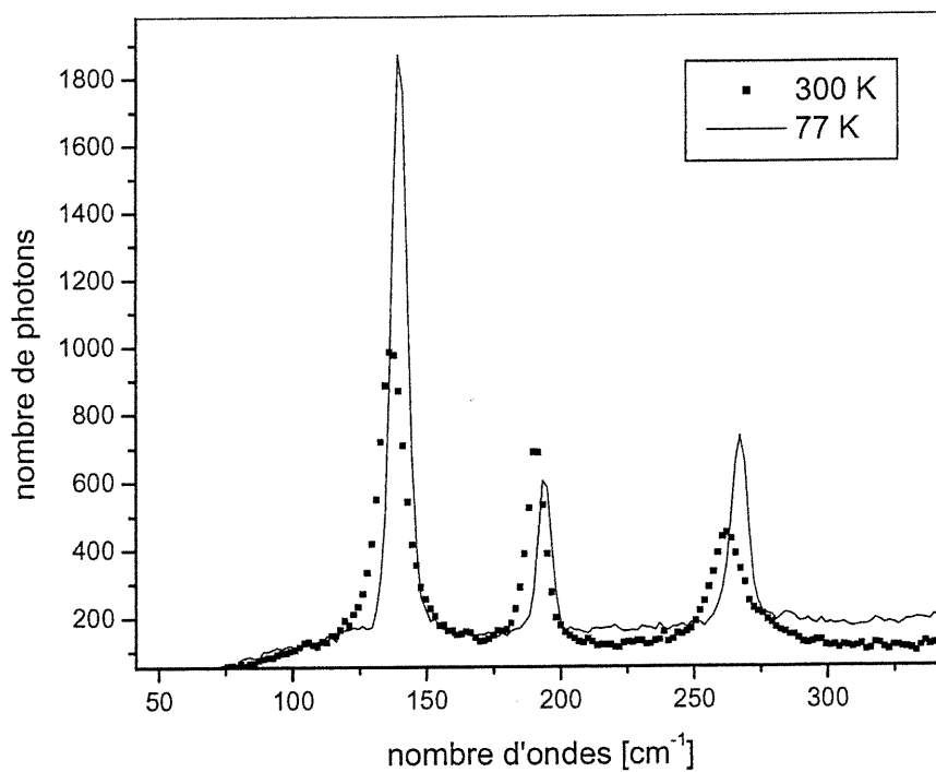
Figure 5.9 : Spectres Raman du composé \text{CsNiCl}_3 en phase solide avec laser 514 nm à différentes températures dans l'orientation perpendiculaire.
