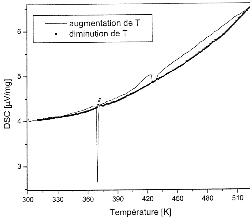
Figure 6.4 : Mesures de DSC du composé \text{Cat}_2\text{Ni}_2(\text{NCS})_8 .
