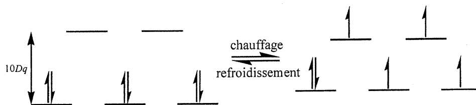
Figure 6.1 : Modification de la structure électronique des composés de fer(II) en coordination octaédrique[7] lors de la transition thermochromique.
