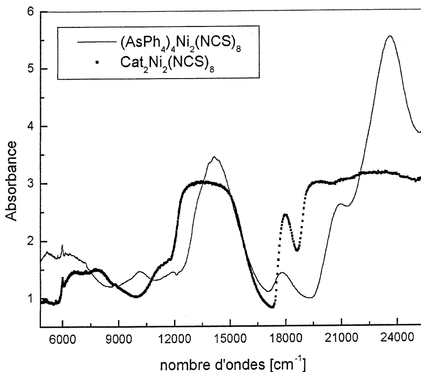
Figure 4.11 : Spectres d'absorption du (\text{AsPh}_4)_4\text{Ni}_2(\text{NCS})_8 et du \text{Cat}_2\text{Ni}_2(\text{NCS})_8 à 5 K.
