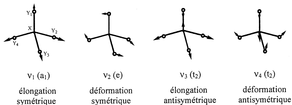
Figure 3.2 : Modes normaux de vibration d'un tétraèdre de type \text{XY}_4 . [12]
