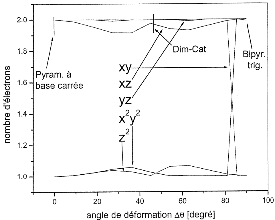
Figure 6.6 : Évolution de la structure électronique des orbitales d de l'état fondamental lors du passage de la pyramide à base carrée (symétrie C_{4v} ) vers la bipyramide trigonale (symétrie D_{3h} ). Voir figure 6.7 pour la signification de angle de déformation \Delta\theta . Pour ce diagramme nous avons utilisé \Delta\phi = \Delta\theta / 3 . Note : Dim-Cat \equiv Cat_2Ni_2(NCS)_8 .
