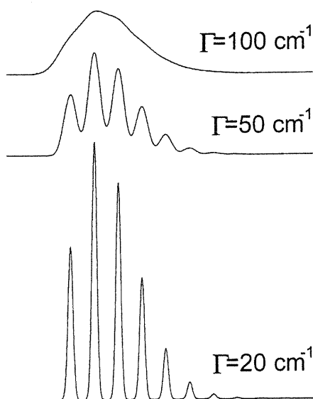
Figure 3.11 : Spectre d'absorption calculé avec différentes valeurs de \Gamma .
