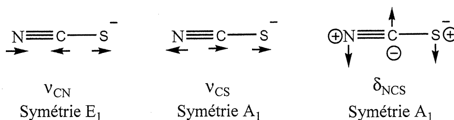
Figure 3.20 : Vibrations centrées sur le ligand \text{NCS}^- .
