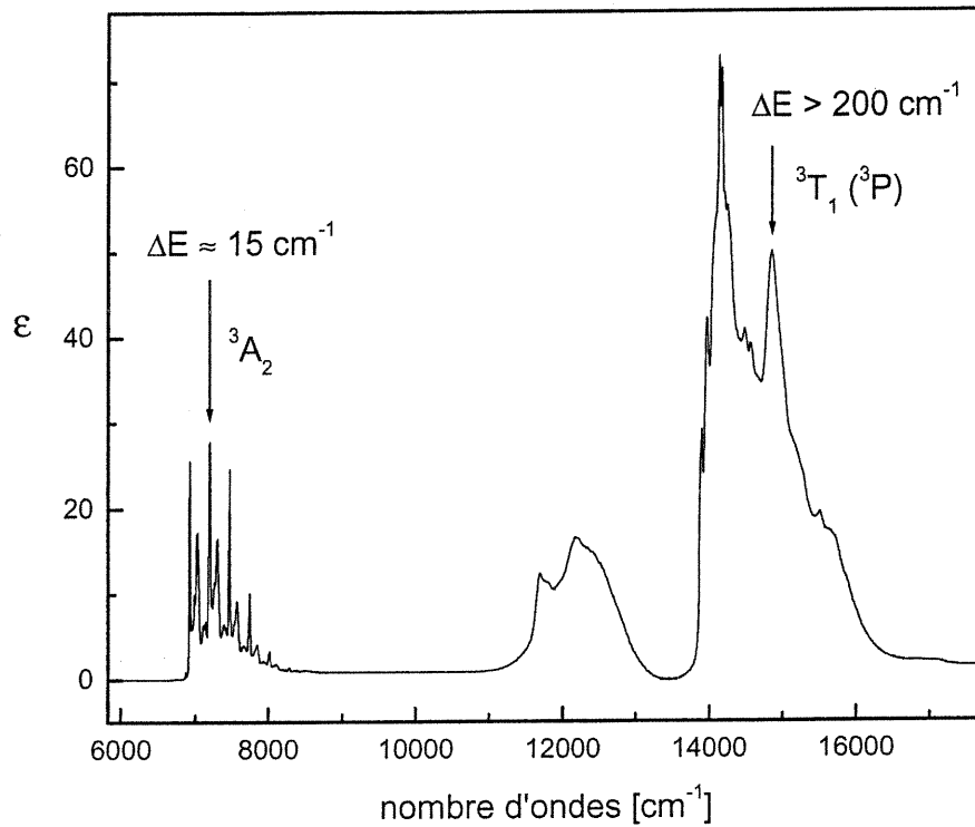
Figure 3.13 : Largeur des pics observés dans le spectre d'absorption du (\text{Et}_4\text{N})_2\text{NiCl}_4 .
