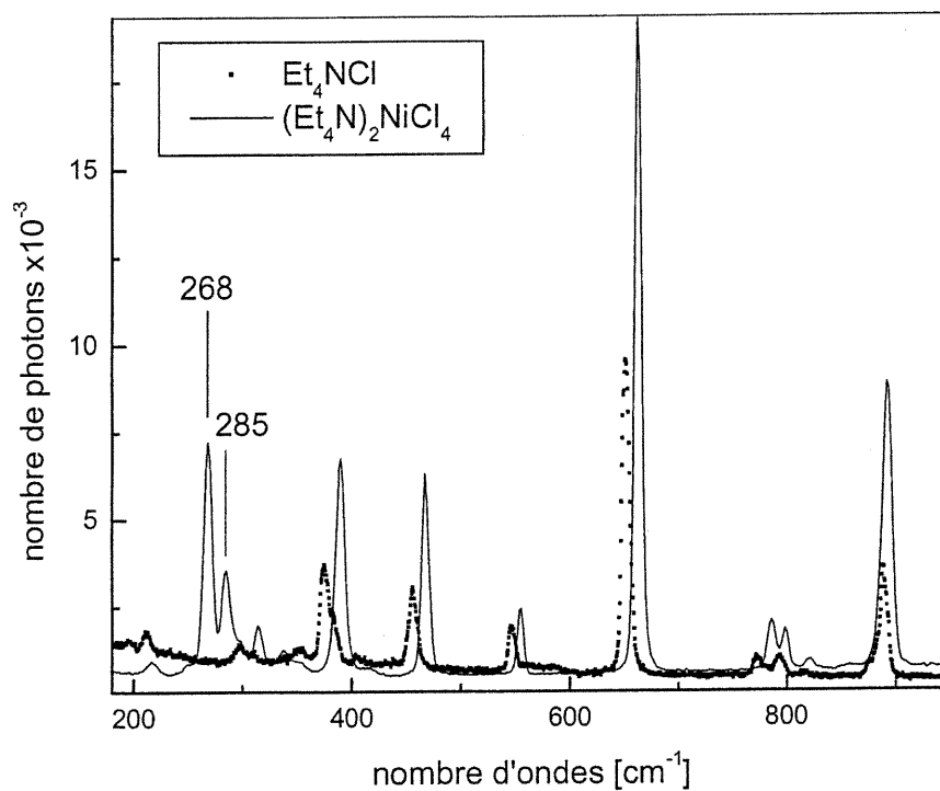
Figure 3.4 : Spectre Raman, à 77 K, du (\text{Et}_4\text{N})_2\text{NiCl}_4 (laser 514 nm) et du \text{Et}_4\text{NCl} (laser 782 nm). Les deux spectres ont été mesurés avec le système Renishaw 3000.
