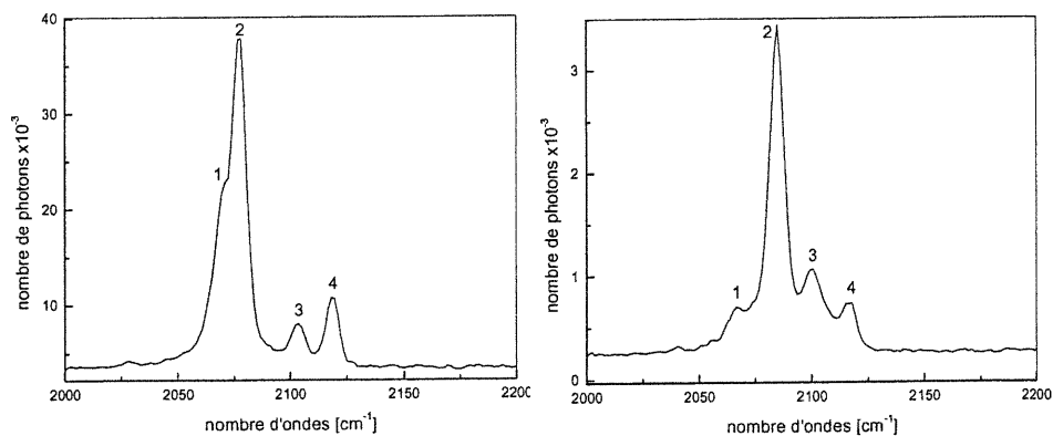
Figure 3.25 : Spectre Raman à 77 K avec laser 514 nm du (\text{AsPh}_4)_2\text{Ni(NCS)}_4 (à gauche) et du \text{CatNi(NCS)}_4 (à droite).
