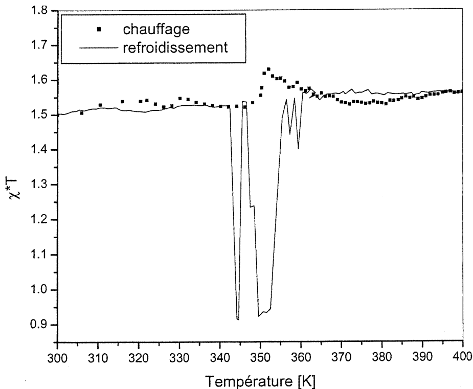
Figure 6.3 : Mesures magnétiques du composé \text{Cat}_2\text{Ni}_2(\text{NCS})_8 dans la région de la transition thermochromique ( \approx 115^\circ\text{C} \equiv 388\text{ K} ).
