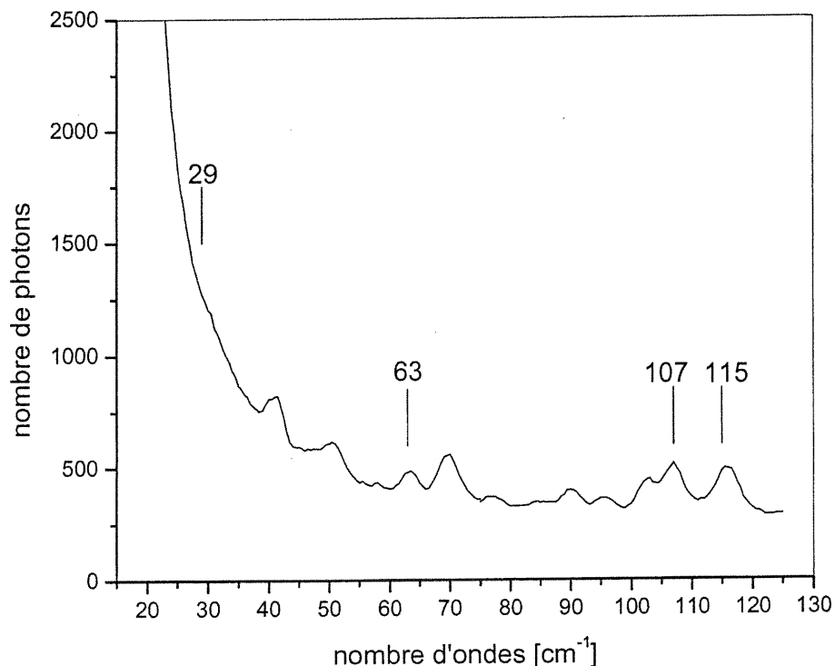
Figure 3.5 : Spectre Raman d'un cristal de (\text{Et}_4\text{N})_2\text{NiCl}_4 à 5 K mesuré avec le monochromateur Spex 14018 avec une longueur d'onde laser de 514 nm.
