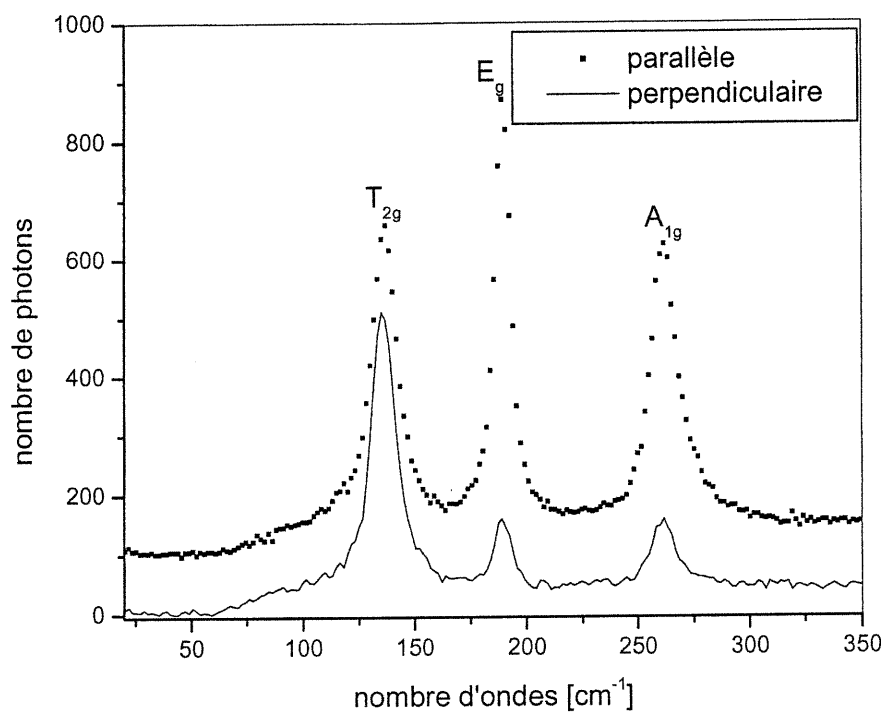
Figure 5.8 : Spectres Raman du composé \text{CsNiCl}_3 en phase solide avec laser 514 nm dans deux orientations différentes.
