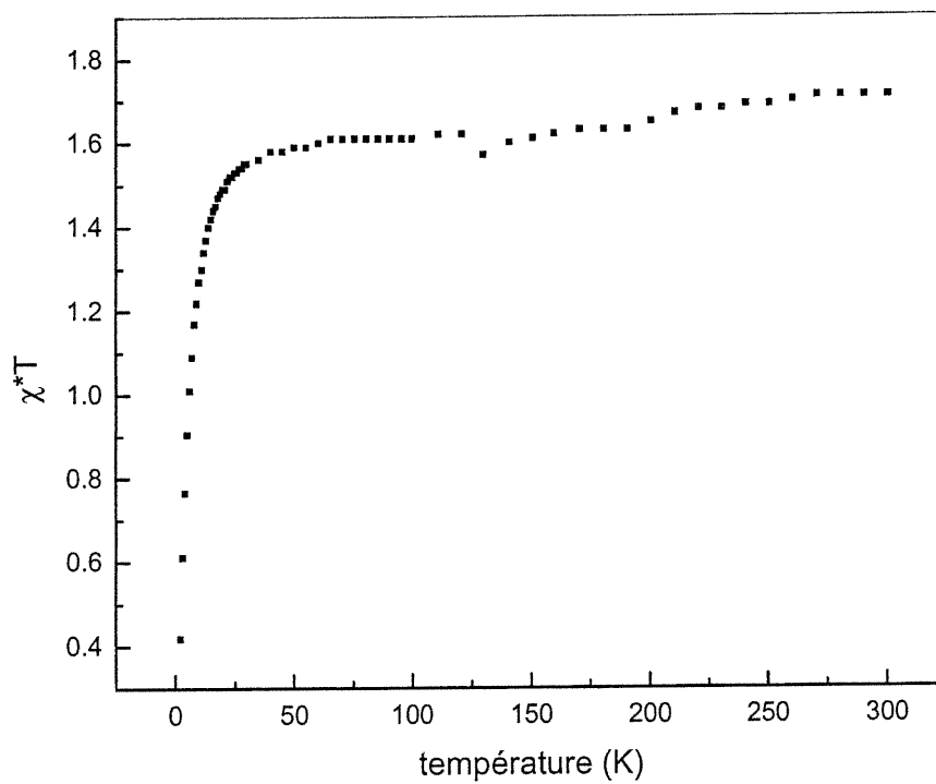
Figure 4.14 : Mesure magnétique pour le composé \text{CatNi}(\text{NCS})_4 .
