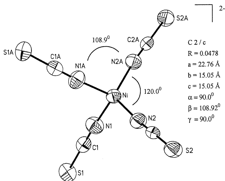
Figure 3.18 : Structure du complexe [\text{Ni}(\text{NCS})_4]^{2-} dans (\text{AsPh}_4)_2\text{Ni}(\text{NCS})_4 à 300 K.
