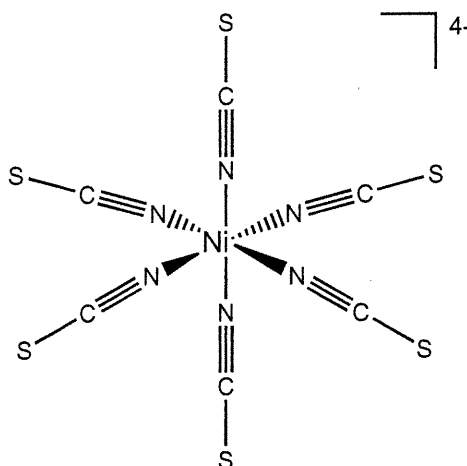
Figure 3.28 : Complexe [\text{Ni}(\text{NCS})_6]^{4-} en coordination octaédrique.
