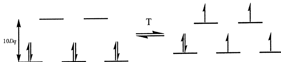
Figure 1.1 : Modification de la structure électronique des composés de fer(II) en coordination octaédrique[7] lors de la transition thermochromique.
