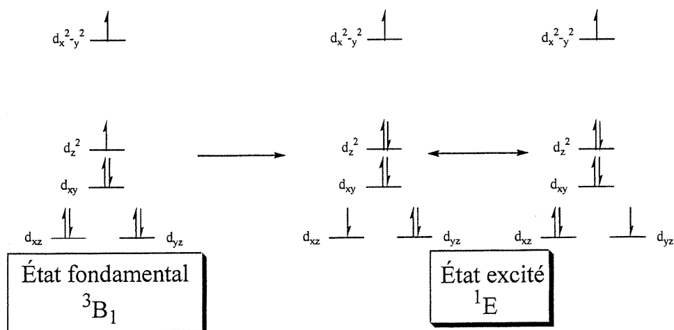
Figure 5.1 : Configurations électroniques de l'état fondamental et d'un état excité pour un complexe de nickel(II) en coordination pyramide à base carré.
