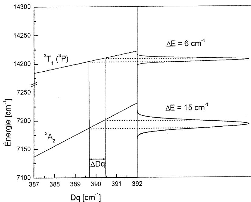
Figure 3.12 : Résolution spectrale et diagramme Tanabe-Sugano.
