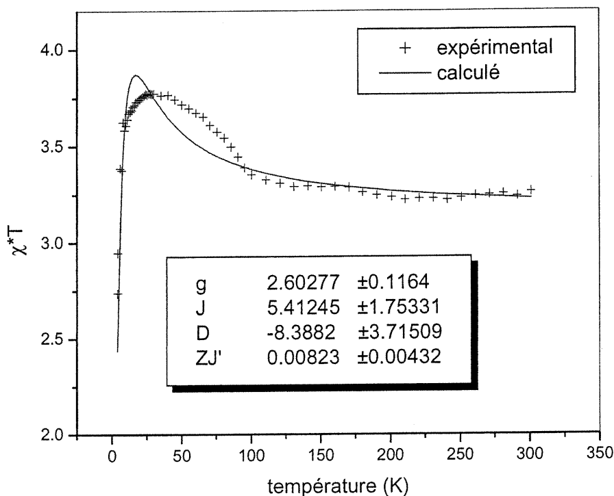
Figure 4.13 : Mesures magnétiques pour le composé \text{Cat}_2\text{Ni}_2(\text{NCS})_8 à basses températures.
