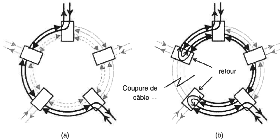
FIG. 2.2 – BLSR 4 fibres (Figure extraite de [Gro03])
