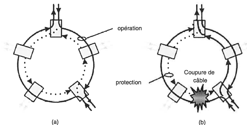
FIG. 2.1 – UPSR (Figure extraite de [Gro03])
