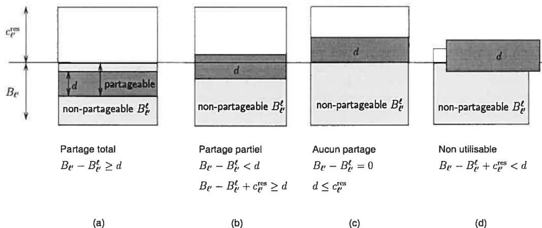
FIG. 3.2 – Bande passante de protection nécessaire sur un lien
