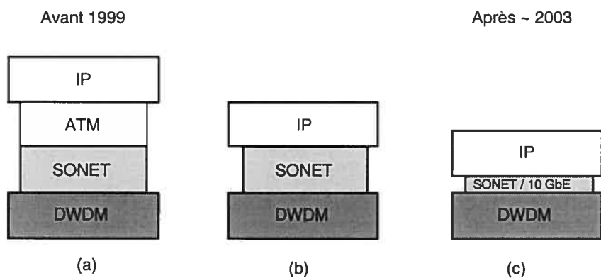
FIG. 1.1 – Les modèles IP sur DWDM
