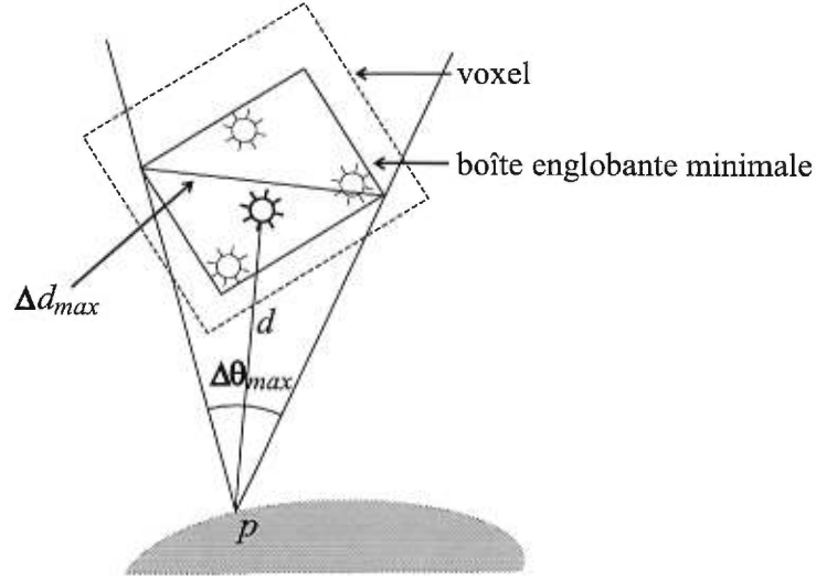
FIG. 5.2: Erreurs maximales des valeurs d et \theta dues à l'utilisation de la hiérarchie.
