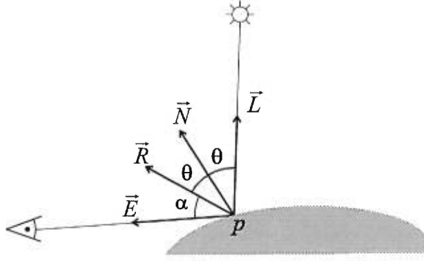
FIG. 2.3: Illustration du modèle de réflexion de Phong.
