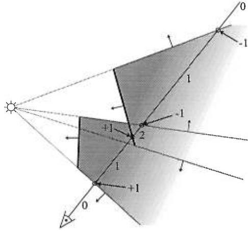
FIG. 3.5: Volume d'ombre déterminé par une source ponctuelle et un polygone. Il est à noter que les normales des polygones d'ombre pointent vers l'extérieur de la zone ombragée.
