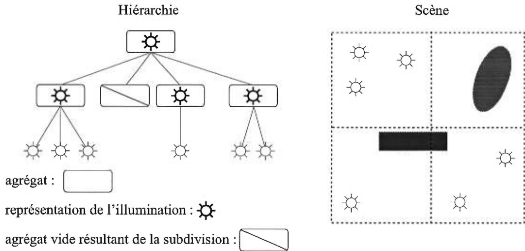
FIG. 4.1: Exemple de représentation hiérarchique de lumières.
