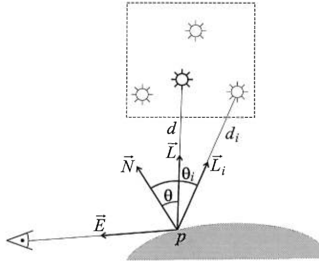
FIG. 5.1: Illustration des différentes valeurs utilisées pour définir la borne d'erreur diffuse.
