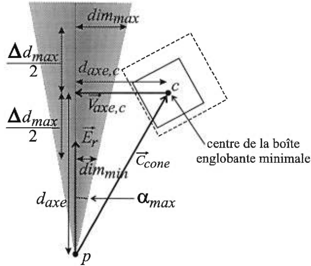
FIG. 5.10: Calcul conservateur de la position d'un voxel par rapport au cône spéculaire.
