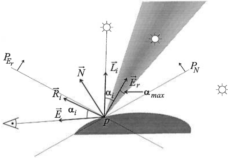
FIG. 5.9: Zone où se trouvent les sources plus importantes pour la réflexion spéculaire.
